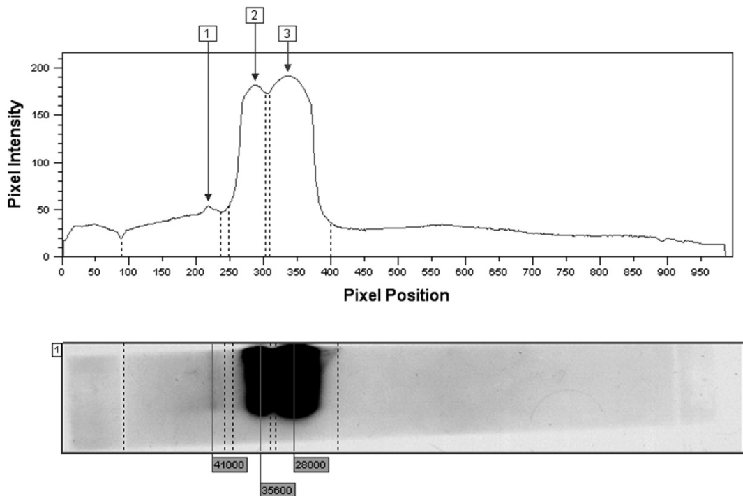
Fig. 6b. Densitogramm of lane 1 Fig. 6a.
